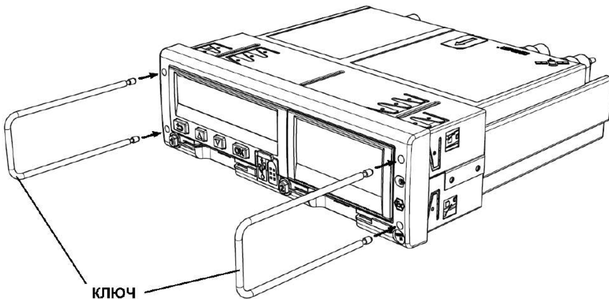
Рисунок 4 – Извлечение тахографа
