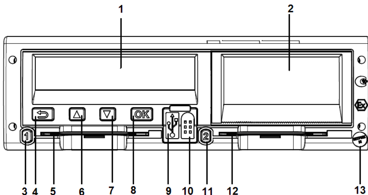
Рисунок 2 – Внешний вид передней панели тахографа
