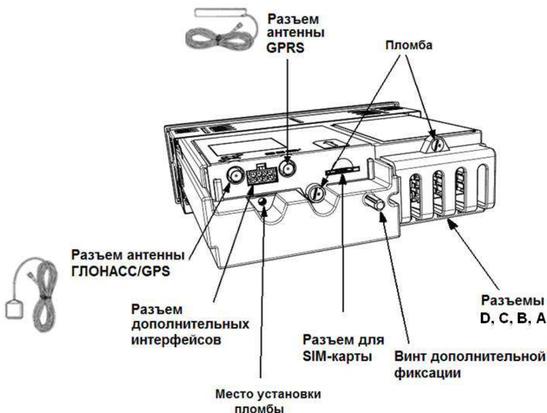
Рисунок 3 – Внешний вид задней панели тахографа
