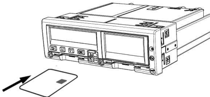
Рисунок 5 – Вставка карты водителя в картоприемник основного водителя «1»
